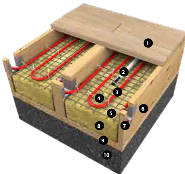
Fig. 13. Trægulv på strøer
