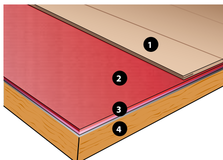
Fig. 17. Gulvvarme med DEVIDry™ på eksisterende undergulv i træ
