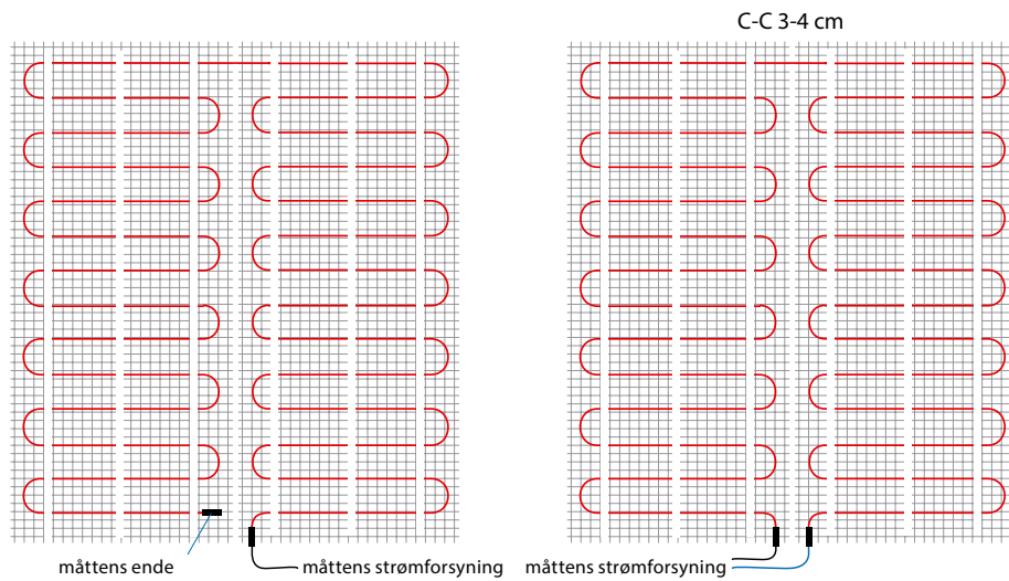
Fig. 7. Eksempel på layout med en varmemåtte med dobbelt- og enkeltleder.
