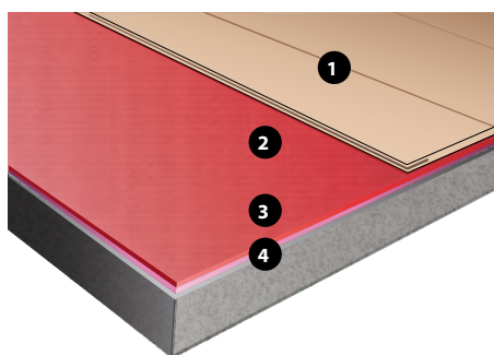
Fig. 16. Gulvvarme med DEVIDry™ på eksisterende undergulv i beton
