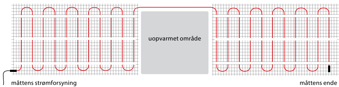
Fig. 8. Layout for en måtte rundt om et uopvarmet område/en forhindring.
