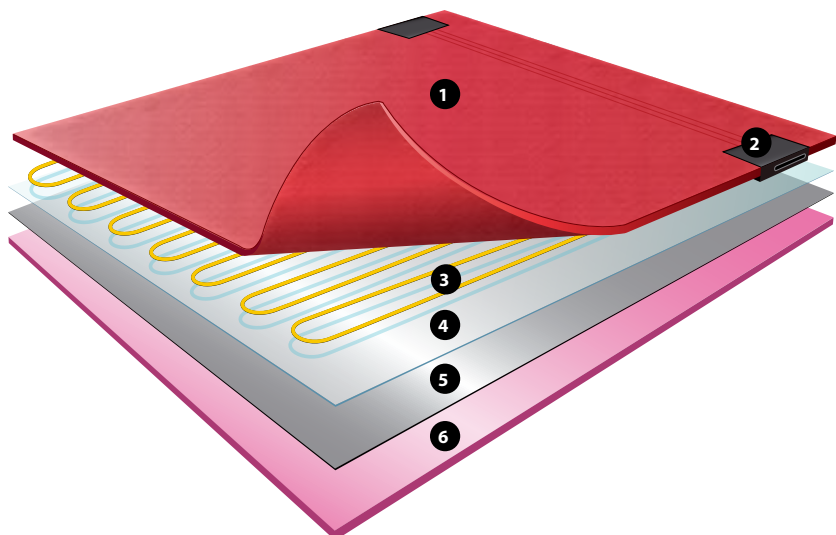
Fig. 15. DEVIDRY™-varmeelementkonstruktion
