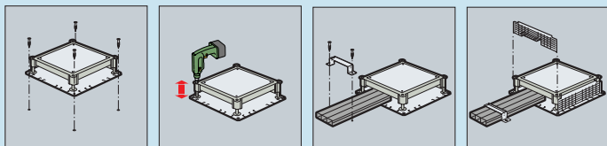
Indstøbning af gulvboks
